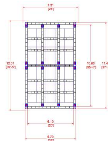
VISTA SUPERIOR
