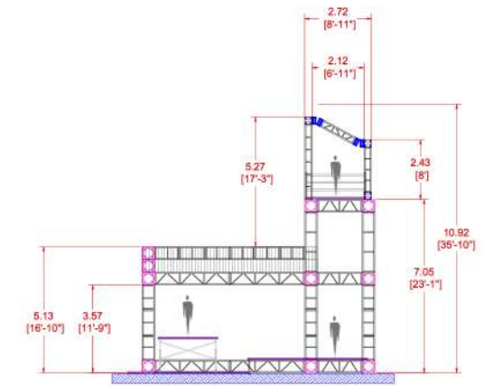
VISTA LATERAL
